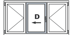
Schéma G 1 vantail coulissant (G ou D) 2 vantaux OF
