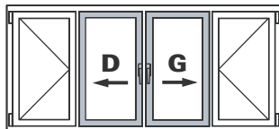
Schéma C 1 vantail coulissant et 1 vantail coulissant semi-fixe (G ou D) 2 vantaux OF
